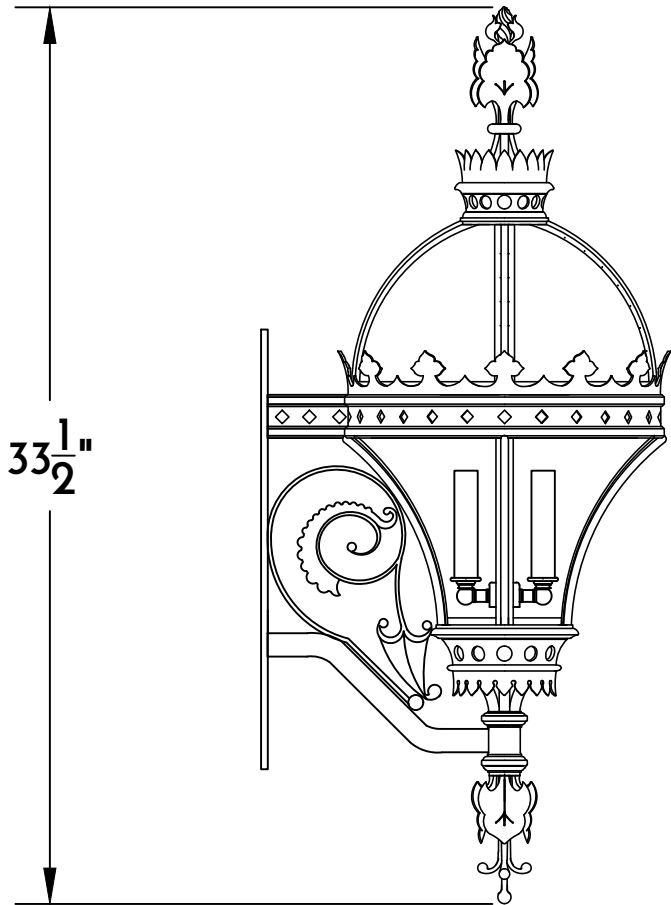
① WALL LANTERN SIDE ELE.
