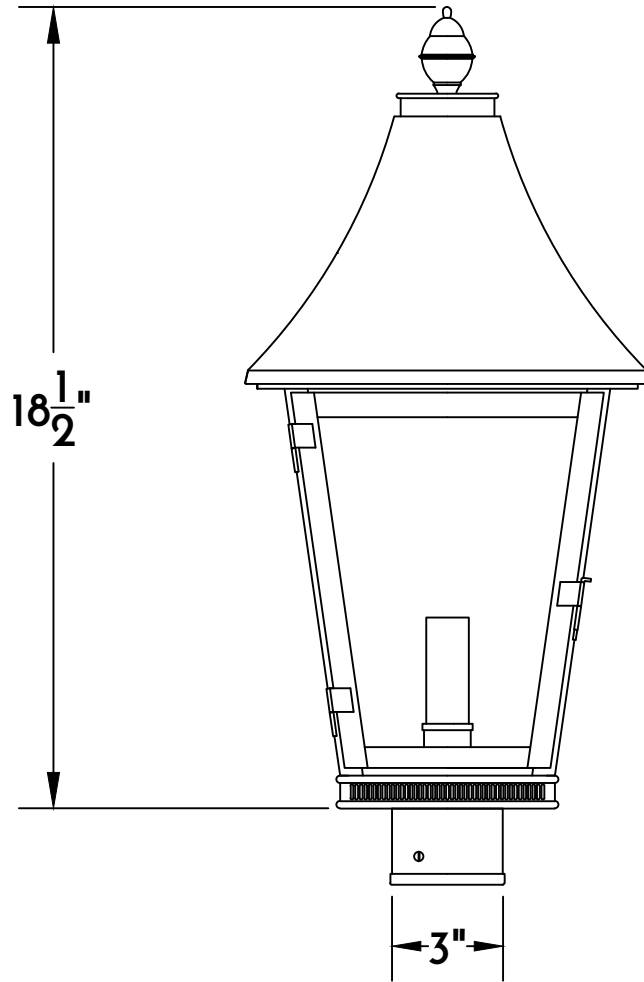
① POST LANTERN SIDE ELE.
