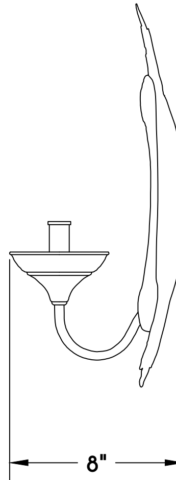
② SCONCE SIDE ELE.
