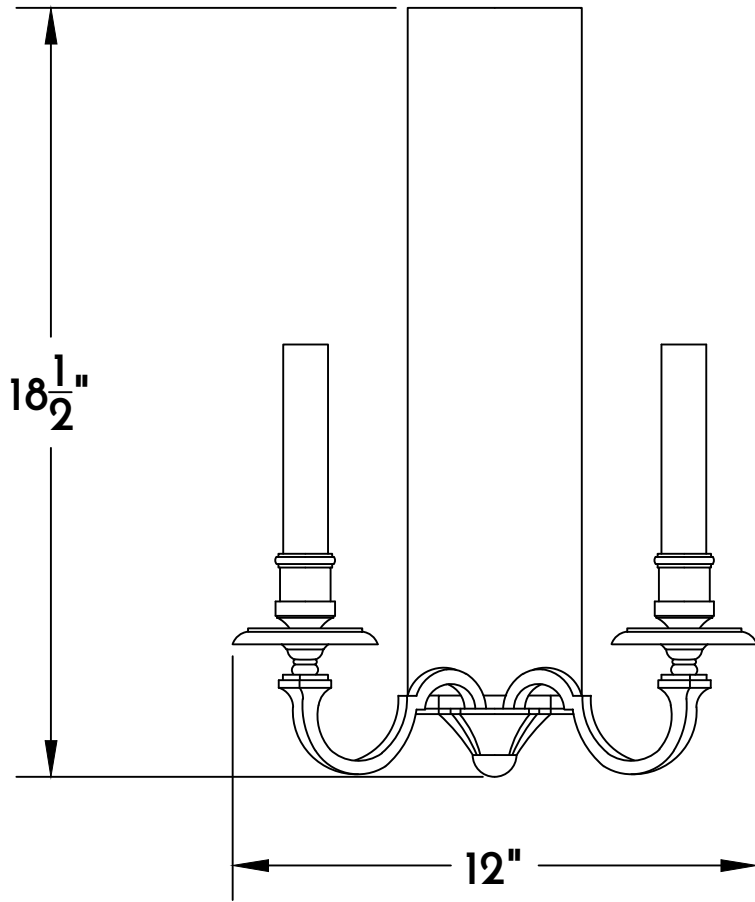
① SCONCE FRONT ELE.
