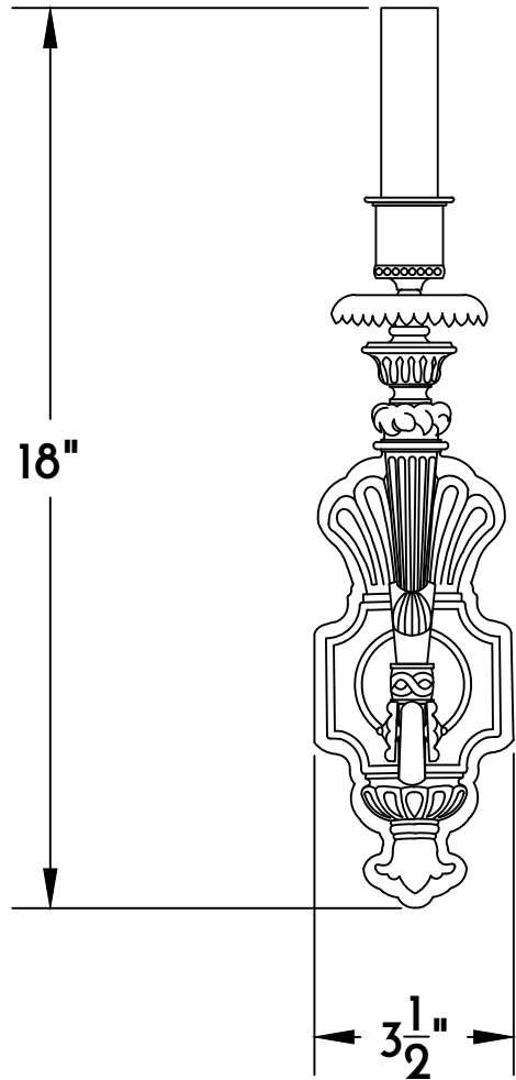
① SCONCE FRONT ELE.
