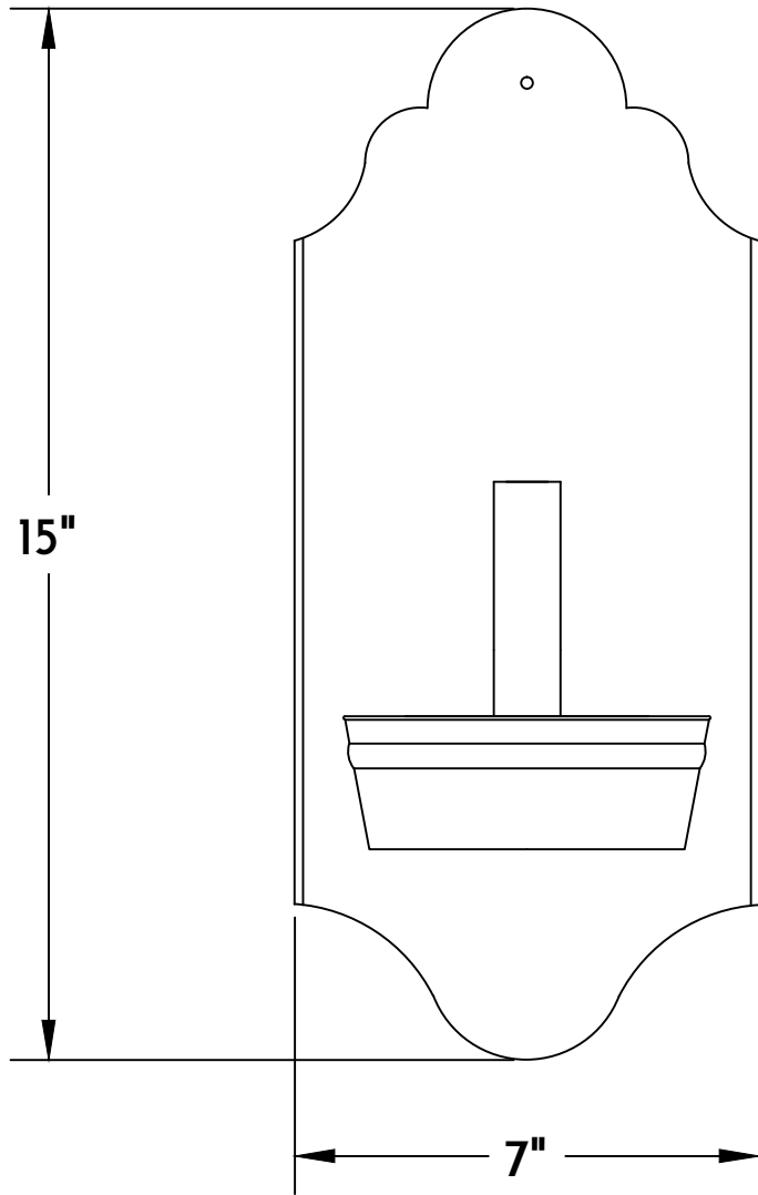
① SCONCE FRONT ELE.
